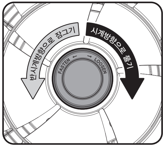
▲시계 방향으로 돌려서 팬 홀더를 제거합니다.
